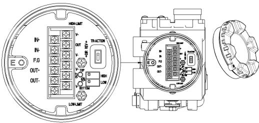
图：接线端子位置
