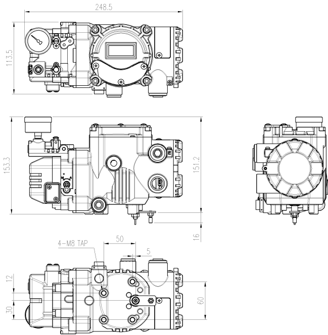
图：YT-3400R 外形图
