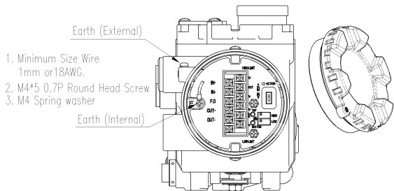
图：接地端子的连接
