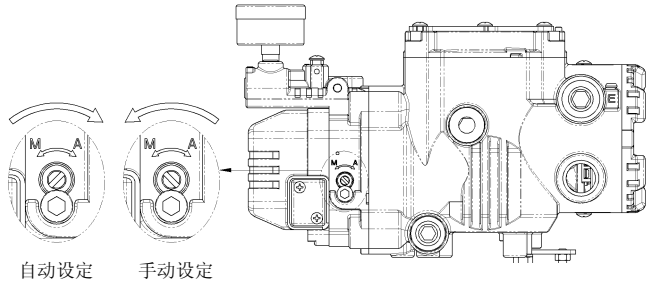
图：自动/手动开关调节
