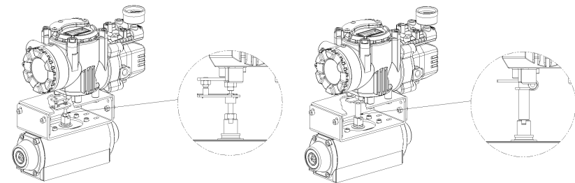
图：利用叉形反馈杆的安装图
