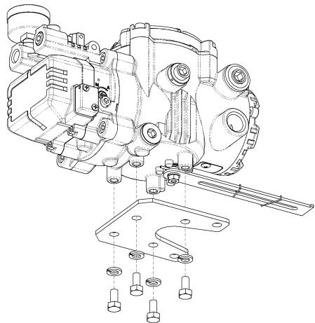
图：YT-3400L 和 支架 连接 图
