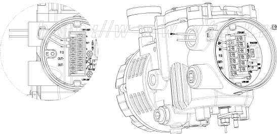
图：电流输入信号端子的连接
