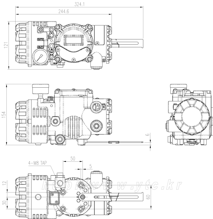
YT-2600L 外形尺寸图
