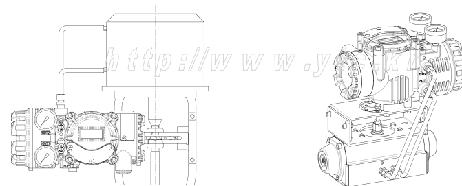
图：双作用执行机构的气管连接例图
