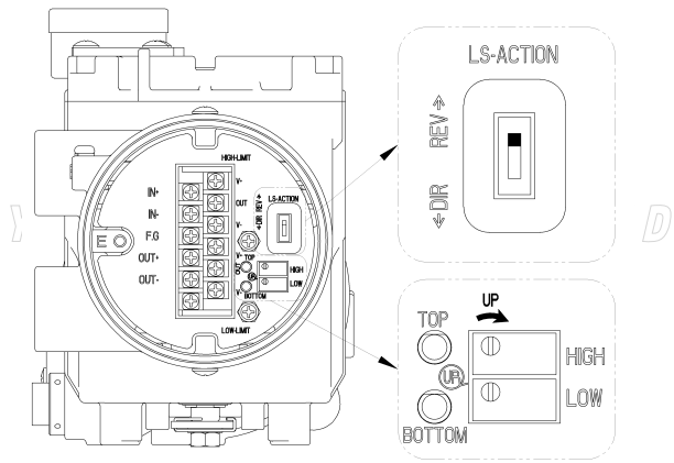
图：限位开关的设定
