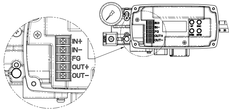
图：YT-2500标准型产品接线图
