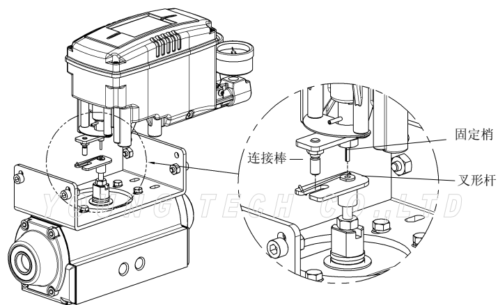
图：YT-2500R主轴上的固定梢和叉形反馈杆孔的连接
