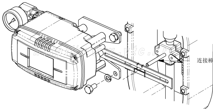
图：阀杆连接件和反馈杆连接
