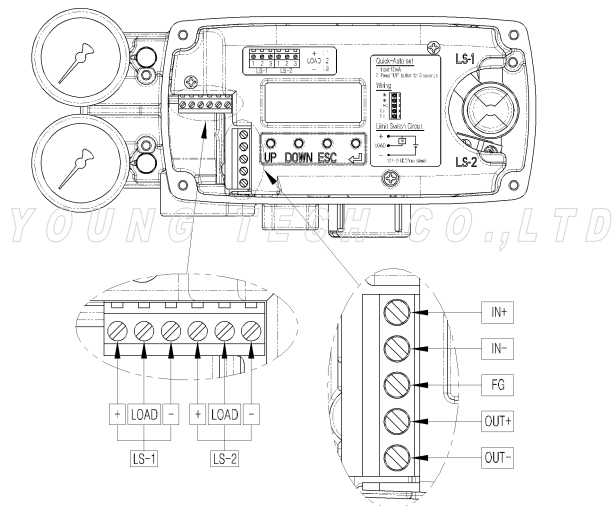
图：内置机械式限位开关接线图
