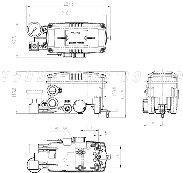
YT-2500R外形尺寸图
