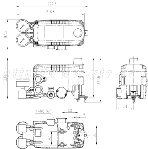
YT-2500R内置限位开关外形尺寸图
