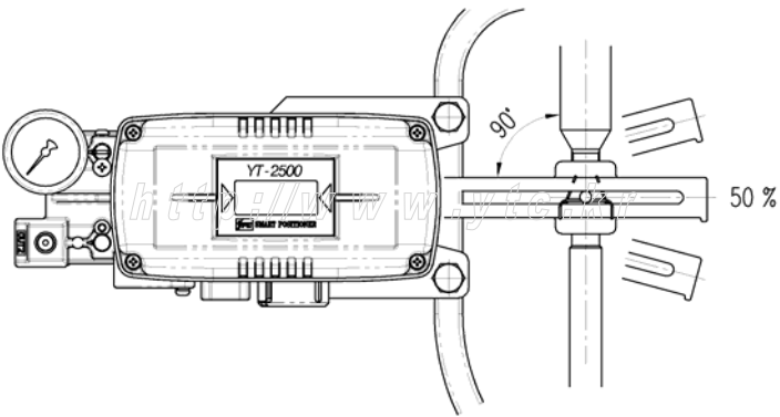
图：反馈杆正确成水平的状态图
