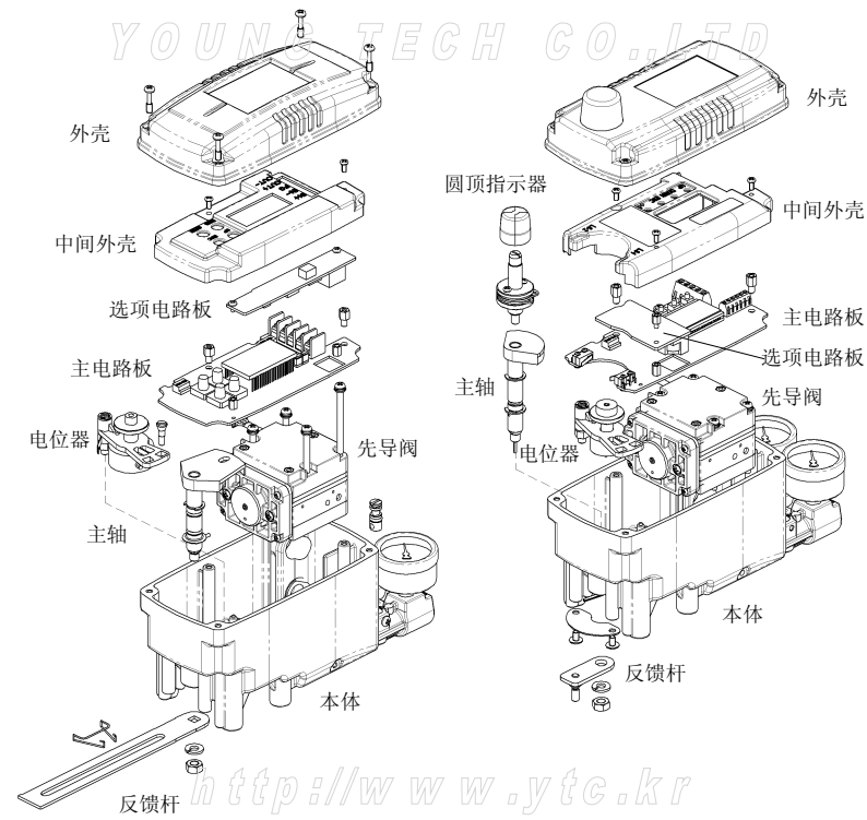
图：YT-2500 内置限位开关结构图
