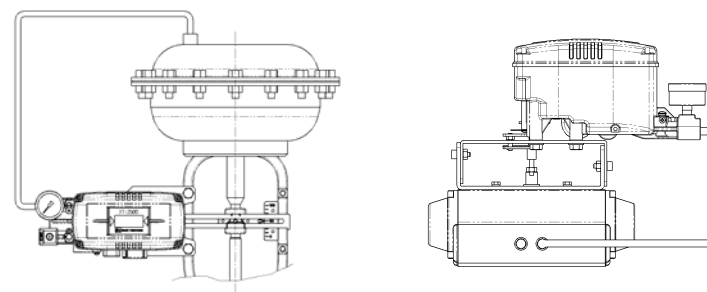
图：单作用执行机构的气管连接例图
