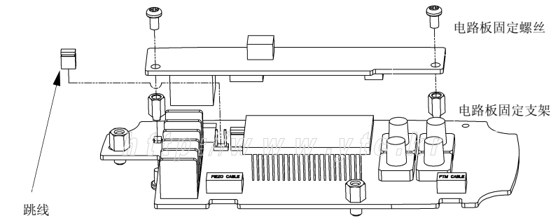
图：选项模块电路板的安装方法
