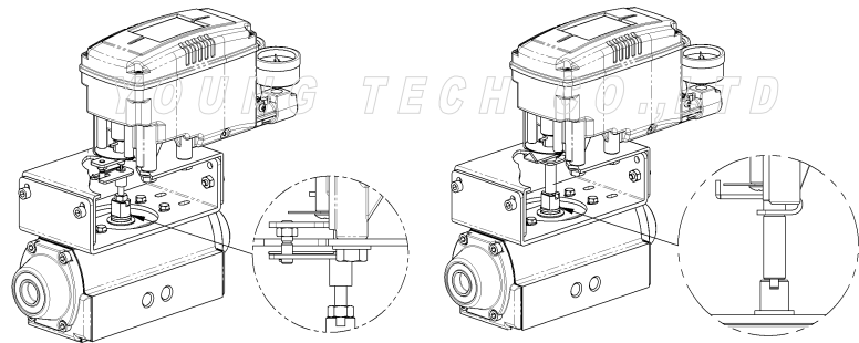
图：利用叉形反馈杆的安装图
