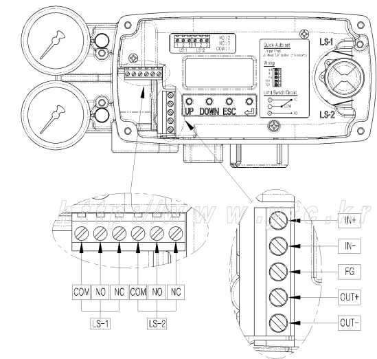
图：内置感应式限位开关接线图
