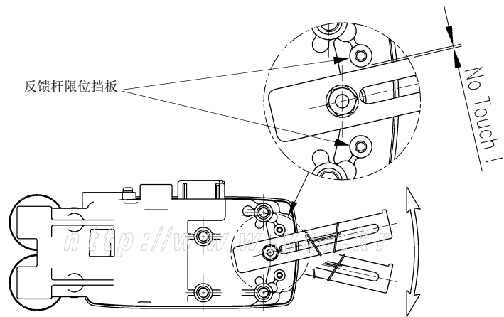
图：反馈挡板和反馈杆之间非接触的状态图
