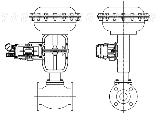
图：YT-2500L 安装例图
