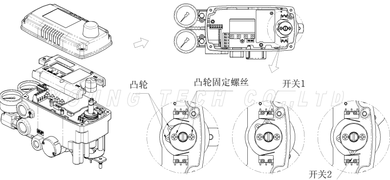
图：机械式限位开关
