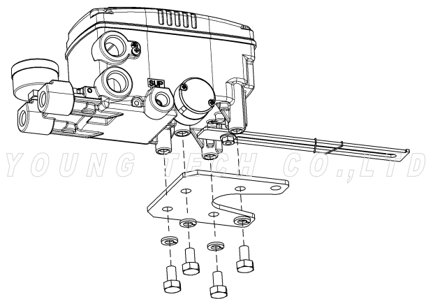
图：YT-2500L 和支架连接图
