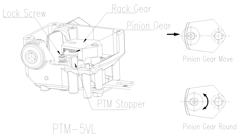
<图12> SPTM-5VL可变电阻位置调整
