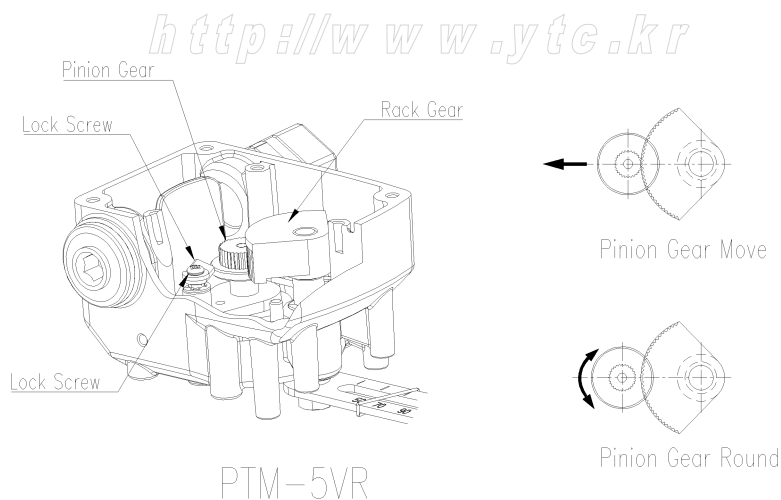
<图13> SPTM-5VR可变电阻位置调整
